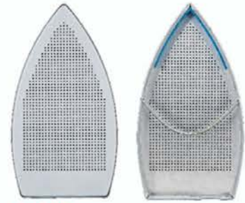
STB-275 41 208×110mm
